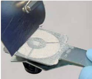
Kleber (Sikadur®-31+) auftragen Apply adhesive (Sikadur®-31+)
